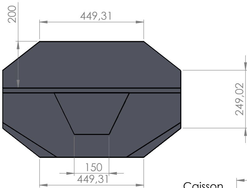
Caisson médium 20TK8R
